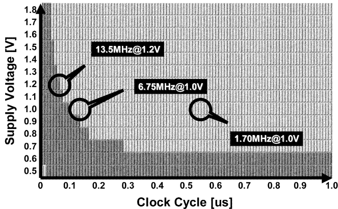
Fig. 21. Shmoo plot.
